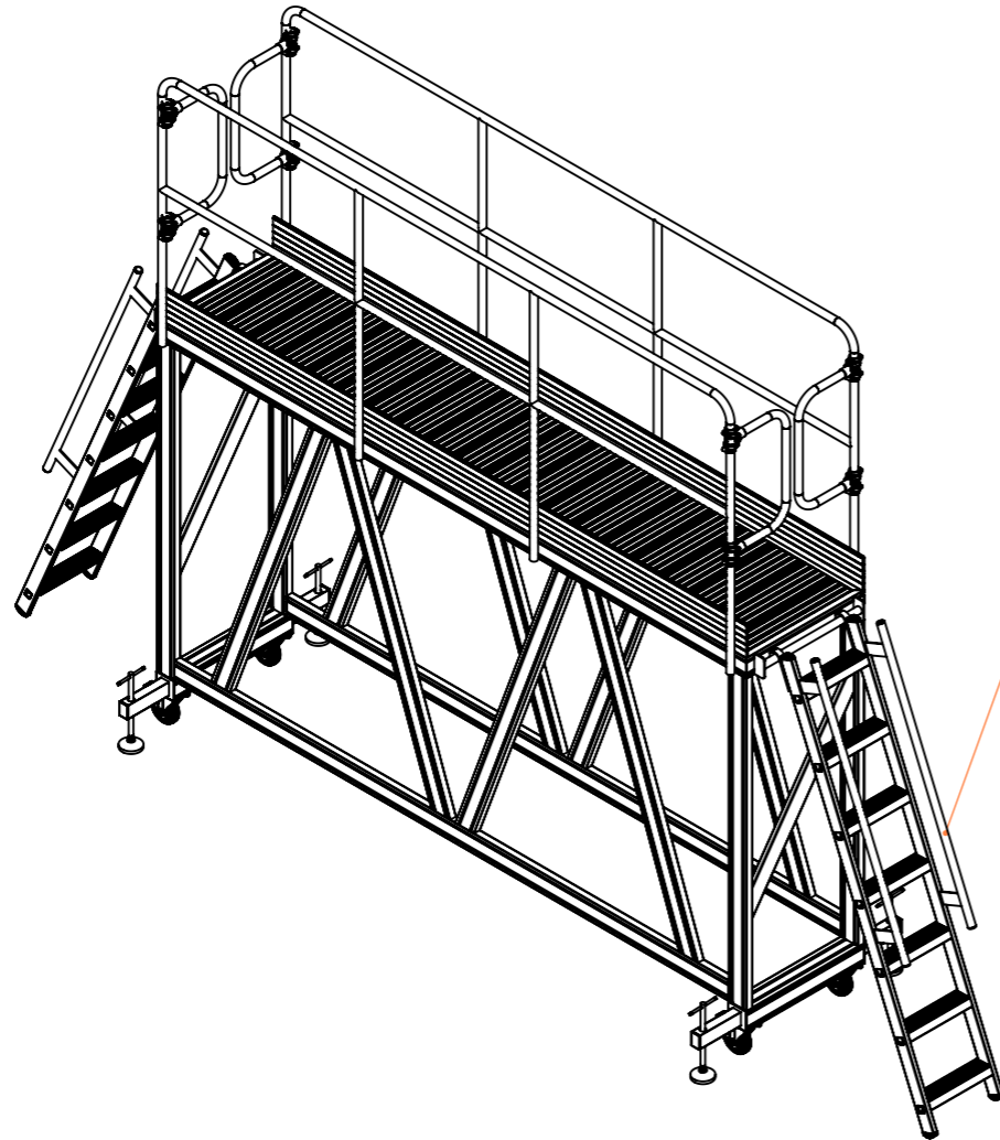
SÖKÜLEBİLİR SEYYAR KORKULUKLU MERDİVEN
